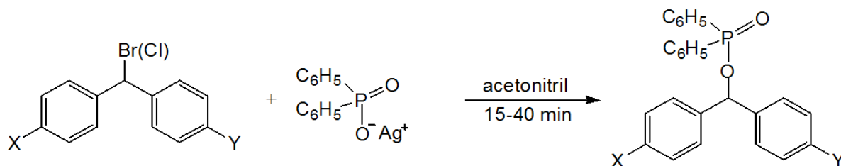
Slika 25. Reakcijska shema sinteze X,Y-supstituiranih benzhidrilnih difenil-fosfinata
