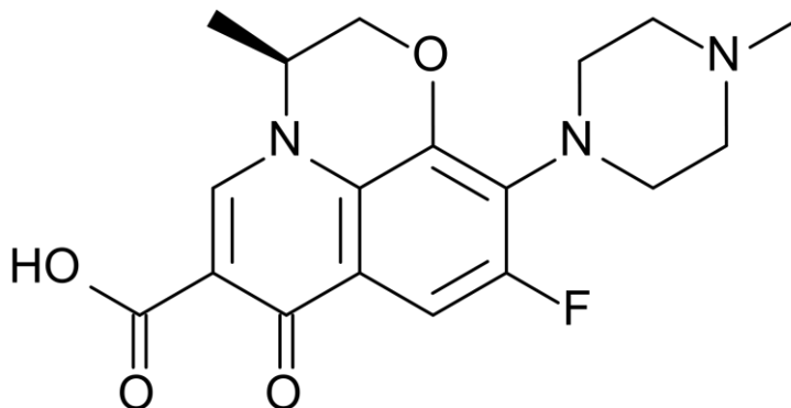
Slika 10. Levofloksacin
