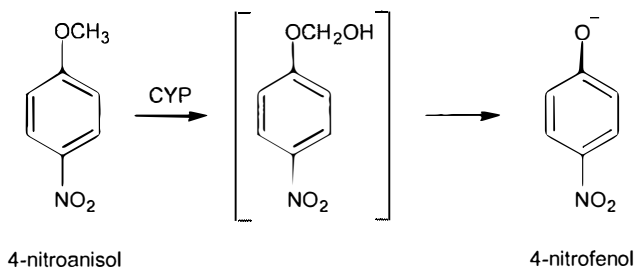
Slika 4. O-demetilacija 4-nitroanisolola
