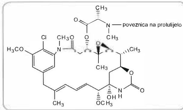
Slika 3. Maitansinoid DM1
