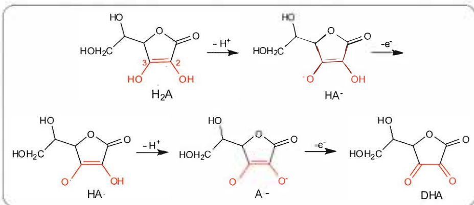
Slika 1. L-askorbinska kiselina ( H_2A ) i njezina oksidacija preko askorbil radikala ( A^\cdot ) u dehidroaskorbinsku kiselinu (DHA).
