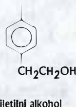
Sl. 5. Najčešće sastavnice eteričnog ulja Pelargonium vrsta
