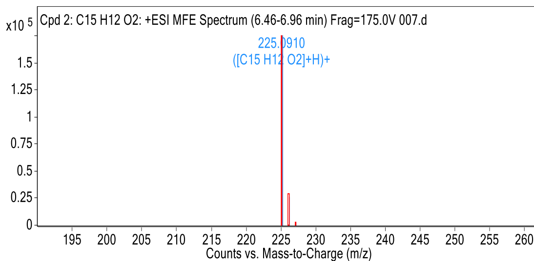
Slika 45. Spektar izdvojenog iona nepoznatog flavonoida ( m/z = 225,0910 ) inkubacijske smjese za 6-hidroksiflavon s dodanim generirajućim sustavom.
