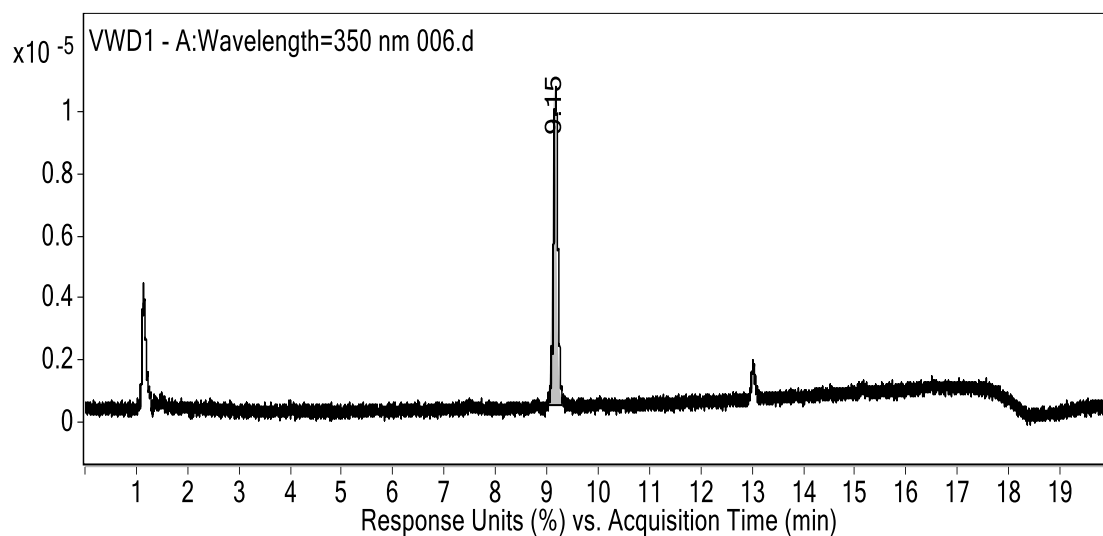
Slika 43. UV kromatogram inkubacijske smjese za 6-hidroksiflavon bez dodanog generirajućeg sustava.
