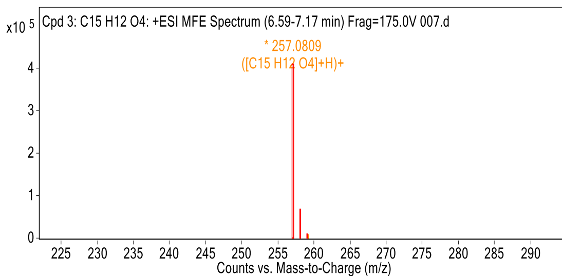
Slika 46. Spektar izdvojenog iona nepoznatog flavonoida ( m/z = 257,0809 ) inkubacijske smjese za 6-hidroksiflavon s dodanim generirajućim sustavom.
