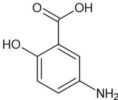
Slika 3. Struktura mesalazina
