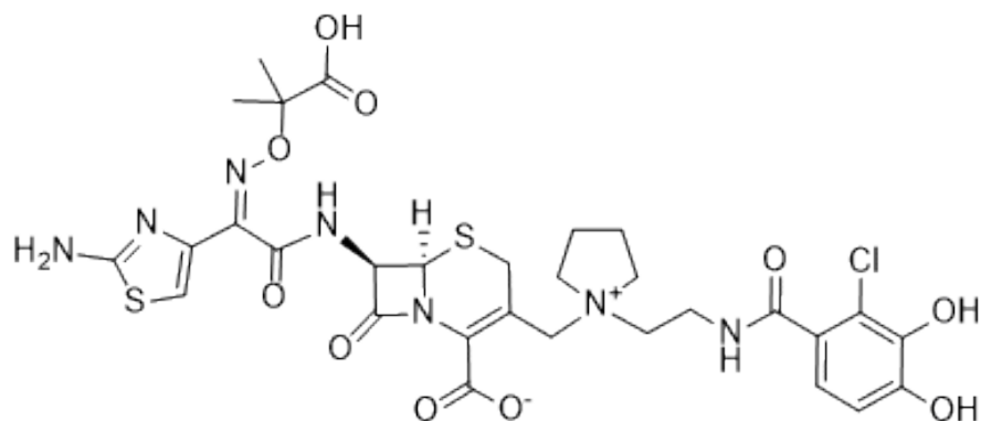
Slika 8. Struktura cefiderokola
