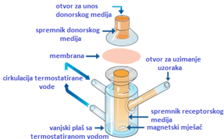
Slika 4. Franz difuzijska ćelija ( www.permeagear.com )
