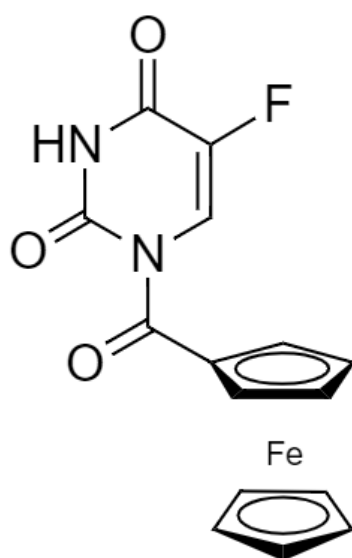
Slika 11. Prikaz N1-ferocenoil-5-fluorouracila
