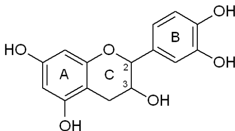
Slika 1.2.1. Struktura (+)-katehina
