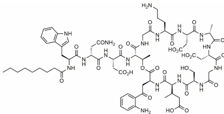
Slika 1. Struktura daptomicina.
