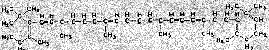
\gamma -karotin
