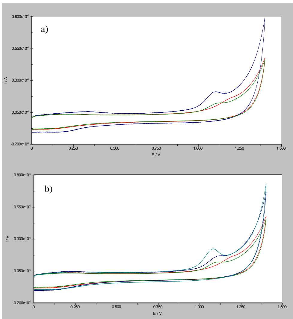
Slika 13. Ciklički voltamogrami pimavanserina u 0,1 M \text{H}_2\text{SO}_4 snimljeni na nemodificiranoj GCE ( c=1\times 10^{-4} M) a) i b) crveno i na GCE modificiranoj različitim nanomaterijalima ( c=5\times 10^{-5} M): GRO a) zeleno, GRNP a) plavo; DNP b) zeleno, CNF b) plavo i GRNT b) tirkizno
