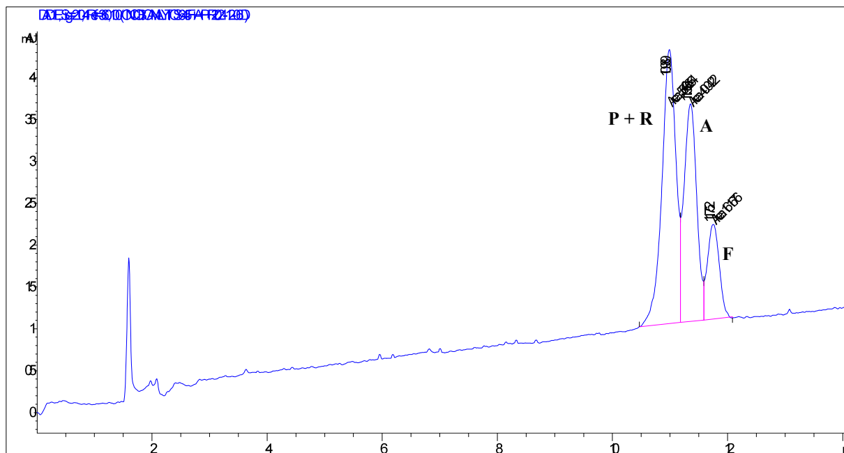
Slika 16. Elektroferogram smjese standardnih otopina fulvestranta, abemacicliba, palbocicliba i ribocicliba.
