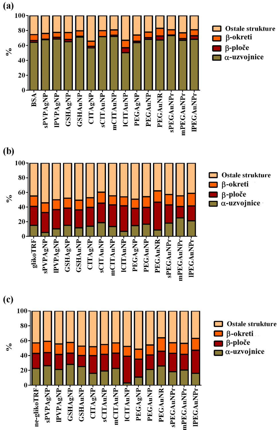
Slika 24. Promjene strukturalnih značajki (a) govedeđ serumskog albumina (BSA), (b) glikoziliranog transferina (glikoTRF) i (c) neglikoziliranog transferina (ne-glikoTRF) uslijed interakcije sa AgNP i AuNP u koncentracijama od 100 \mu M u usporedbi s nativnom konformacijom proteina u ultračistoj vodi pri 25 ^{\circ} C.
