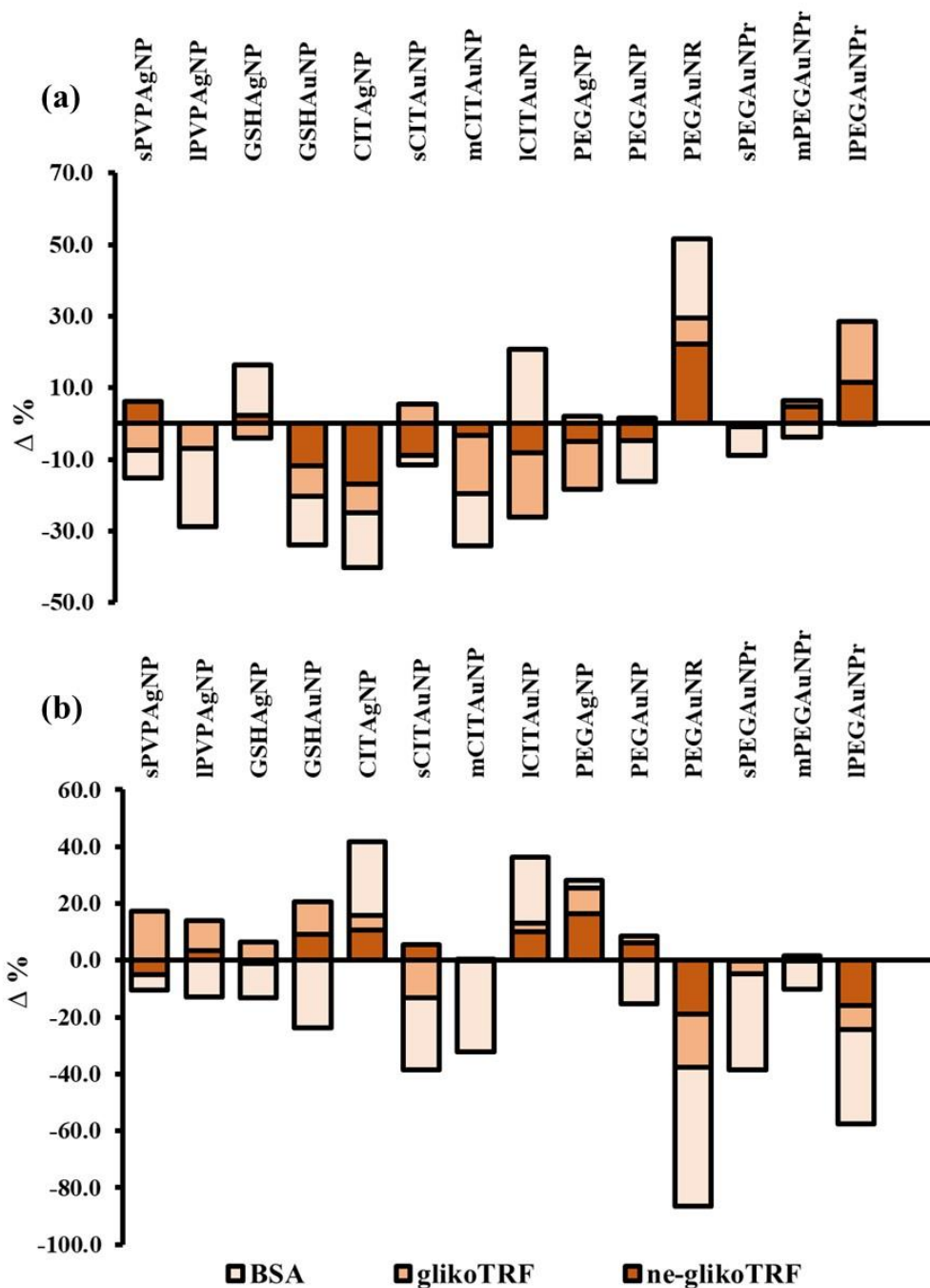
Slika 26. Postotak promjena u (a) \beta -okretima i (b) ostalim strukturama formi goveđeg serumskog albumina (BSA), glikoziliranog transferina (glykoTRF) i neglikoziliranog transferina (ne-glikoTRF) uslijed njihove interakcije sa različitim AgNP i AuNP u koncentracijama od 100 \mu M. Rezultati su dobiveni na koncentracijama proteina od 10 \mu M u ultračistoj vodi pri 25 ^{\circ} C i uspoređeni su sa strukturama nativnih proteina.
