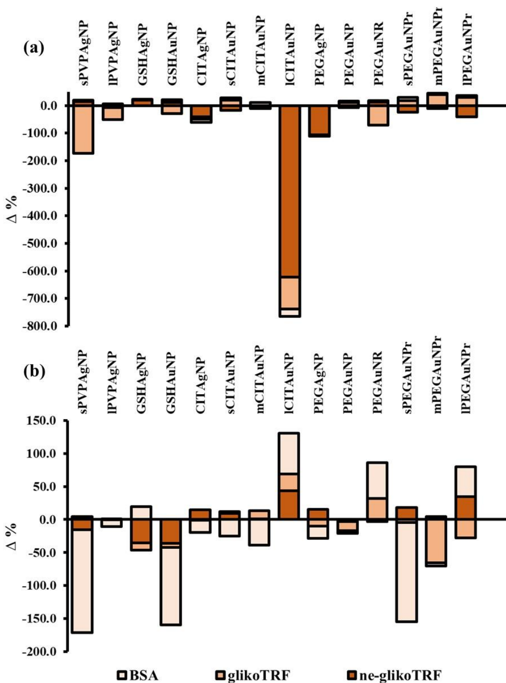
Slika 25. Postotak promjena u (a) \alpha -uzvojnica i (b) \beta -pločama struktura goveđeg serumskog albumina (BSA), glikoziliranog transferina (glykoTRF) i neglikoziliranog transferina (ne-glykoTRF) uslijed njihove interakcije sa različitim AgNP i AuNP u koncentracijama od 100 \mu\text{M} . Rezultati su dobiveni na koncentracijama proteina od 10 \mu\text{M} u ultračistoj vodi pri 25 ^{\circ}\text{C} i uspoređeni su sa strukturama nativnih proteina.
