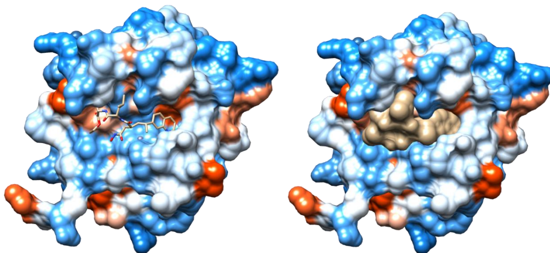
Slika 20. Prikaz hidrofilne/hidrofobne površine proteina 2TCL u kompleksu s ligandom 241 (najuspješniji ligand prvog kruga molekuskog sidrenja). Hidrofobne aminokiseline su označene crvenom bojom, hidrofilne plavom bojom, a neutralne bijelom (izrađeno pomoću programa UCSF Chimera 1.6).
