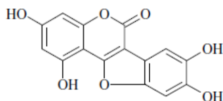
Desmetilvedelolakton
