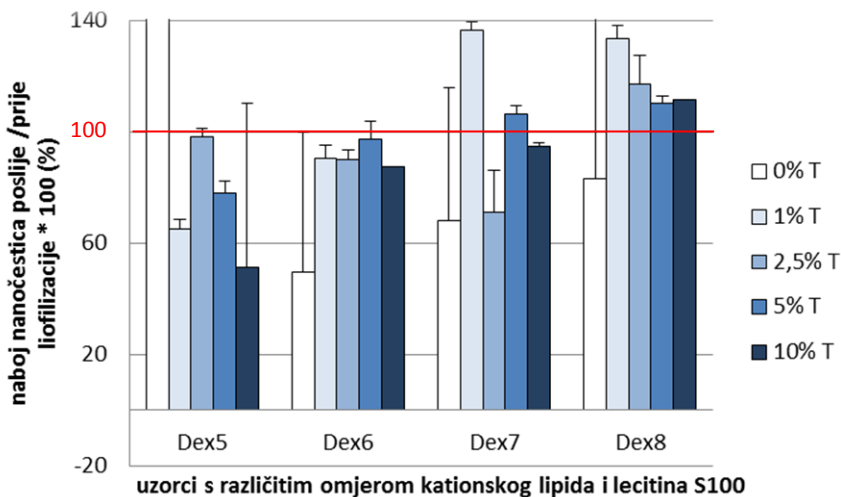
Slika 12. Stupanj očuvanja zeta-potencijala lipidno-alginatnih nanočestica pripremljenih s lecitinom S100 liofiliziranih u prisustvu
