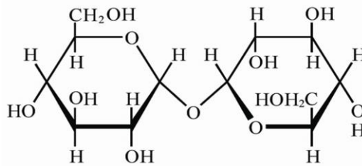
Slika 7. Trehaloza
