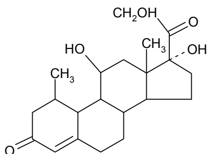
Slika 1.11 Struktura hidrokortizona
