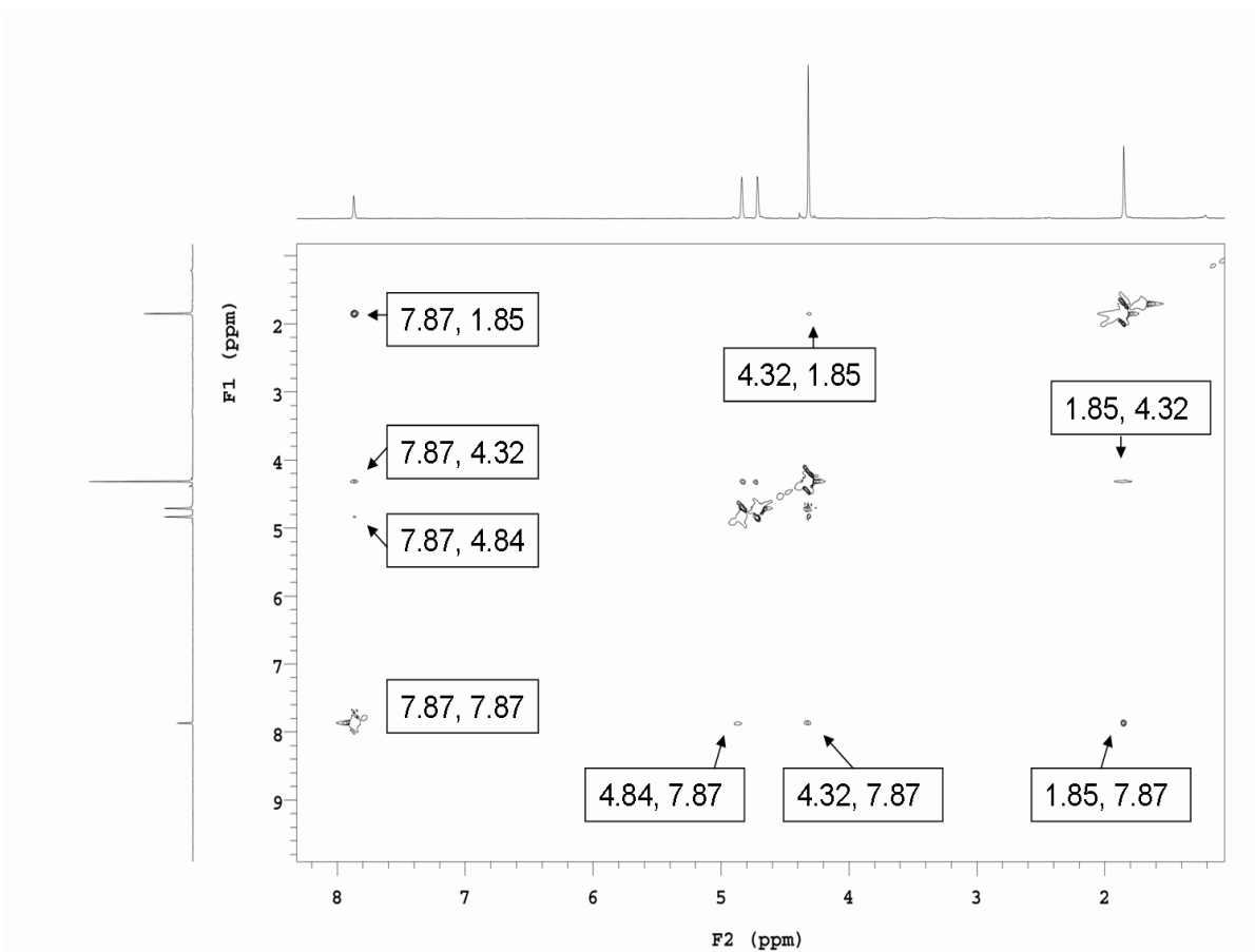
Slika 14. Prikaz NOESY korelacija između određenih vodikovih atoma N1-ferrocenil timina 7b .
