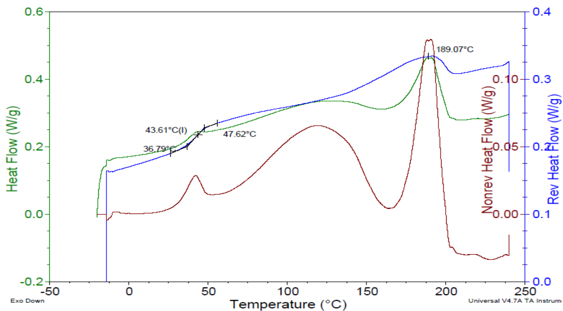
Slika 10. DSC termogram ishodnog polimera PVA 18-88
