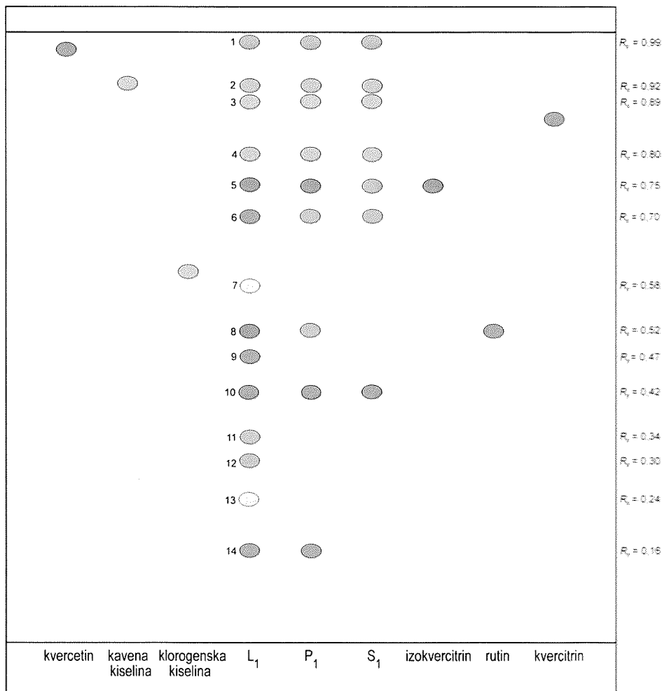
Slika 3. Kromatogram flavonoida i fenolnih kiselina uzorka 1 vučje stope
