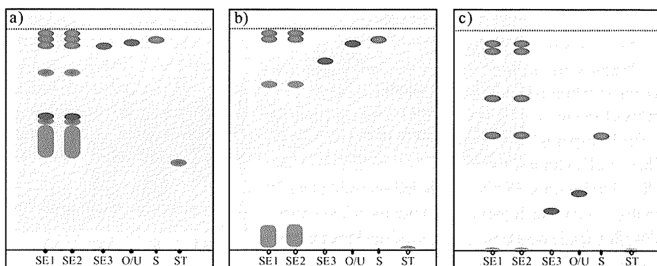
Slike 7a.–c. Kromatogrami saponina, sterola i triterpena ekstrakata korijena primorskog omana (SE1–3) i poredbenih supstancija: saponinskog standarda (ST), stigmasterola/β-sitosterola (S) i oleanolne/ursolne kiseline (O/U) u pokretnim fazama: a) kloroform-metanol-voda (64:50:10 V/V/V), b) kloroform-metanol-voda (80:20:1,5 V/V/V) i c) benzen-aceton (9:1 V/V)
