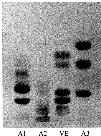
Slika 6. Kromatogram vodenog ekstrakta korijena primorskog omana (VE) i poredbenih aminokiselina A1 (Asp, Ala, Pro, Tyr, Cys), A2 (Lys, Gly, Glu, Met, Phe) i A3 (His, Thr, Val, Leu)
