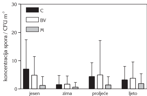
Slika 6 Sezonske varijacije u koncentracijama Fusarium vrsta u zraku na području Zagreba tijekom 2002./03.; u centru grada (C), u Farmaceutskom botaničkom vrtu (BV) i na Medvednici (M)
