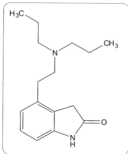
Slika 7. Ropinirol
