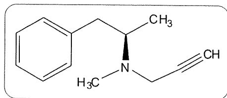
Slika 9. Selegilin
