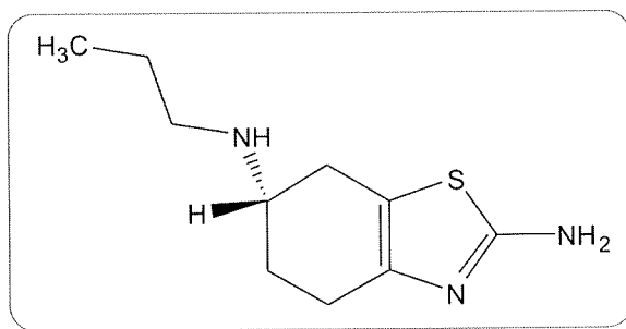
Slika 8. Pramipeksol
