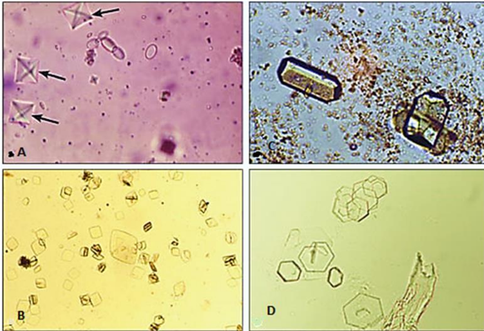
Slika 1. A) kristali kalcijevog oksalata povećanje 100 puta (oblik pisma), B) kristali mokraćne kiseline povećanje 100 puta, C) kristali trip fosfata (oblik lijesa) povećanje 400 putai amornog fosfata, D) kristali cistina povećanje 100 puta (oblik šesterokuta), Urynalisis: A Comprehensive Review, Simerville i sur.
