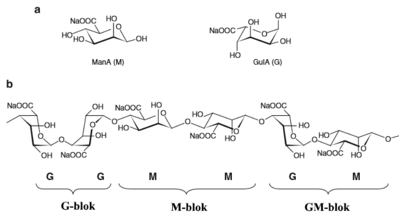
Slika 7: Struktura alginata (preuzeto i prilagođeno prema Rehm, 2009)
