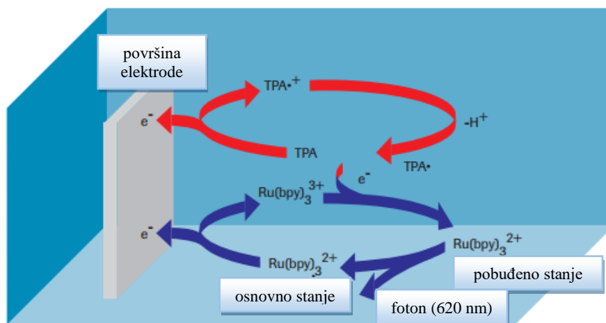
Slika 4. Elektrokemiluminiscentna reakcija na površini elektrode (preuzeto i prilagođeno s http://www.unitedlabs.com.kw/sopdoc/training_files/cobas/cobas.pdf )
