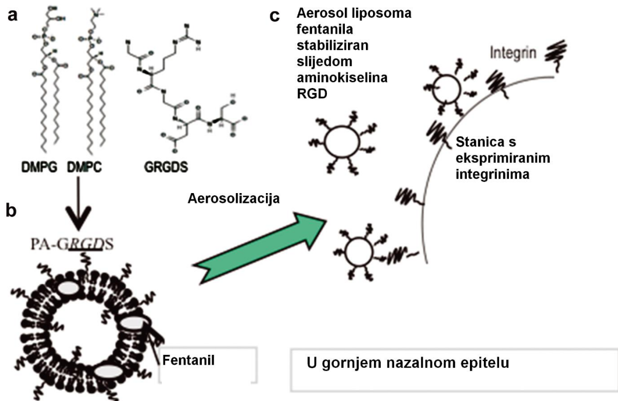
Slika 33. Pregled RGD liposoma i interakcije sa stanicom. (a) Liposom je pripremljen iz smjese 1:1 fosfolipida DMPC i DMPG (DMPC -1,2-dimiristoil-sn-glicero-3-fosfatokolin, DMPG -1,2-dimiristoil-sn-glicero-3-fosfatoglicerol) sa slijedom aminokiselina GRGDS povezanim s palmitinskom kiselinom. (b) Formirani liposom s PA (palmitinskom kiselinom) ugrađenom u dvosloj koja izlaže GRGDS peptid u vanjski okoliš (c) RGD liposomi koji su prikazani u ovoj studiji imaju povećano vezanje na stanice s ekprimiranim integrinima. RGD liposomi su pogodni za dostavu lijeka putem aerosola. (75).
