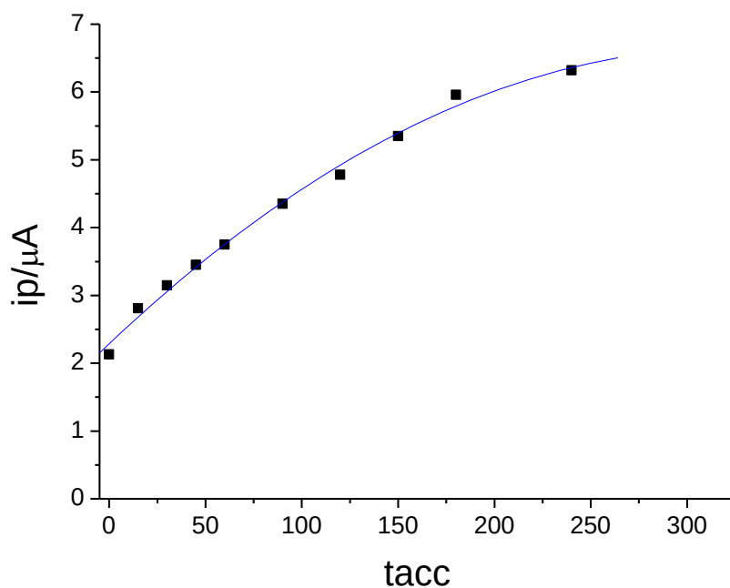
Slika 16. Grafički prikaz ovisnosti izmjerenog strujnog vrha nepafenaka koncentracije 5 \times 10^{-6} M o vremenu akumulacije kod stripping SWV.
