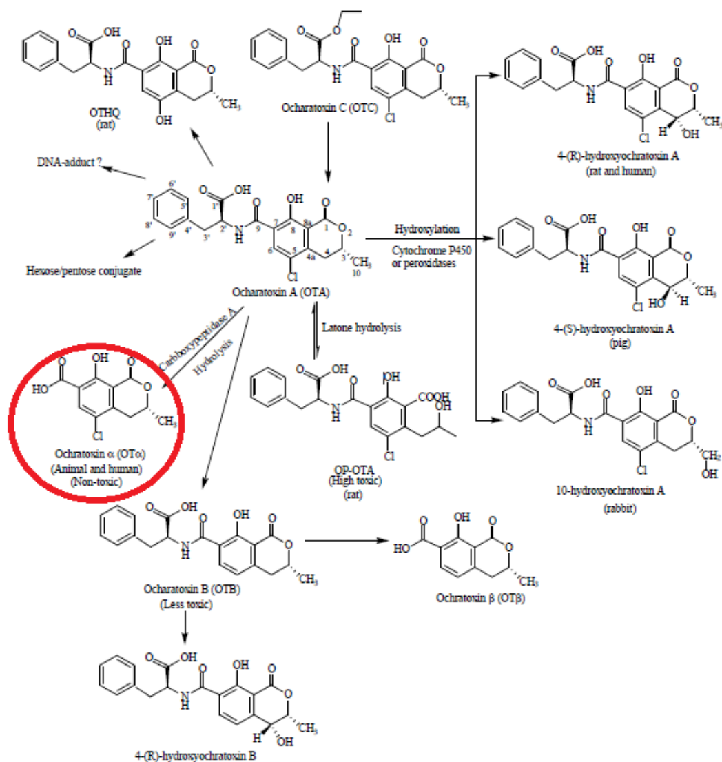
Slika 2. Predloženi metabolički put OTA u životinja i ljudi s crveno zaokruženim najčešćim metabolitom OT \alpha .
