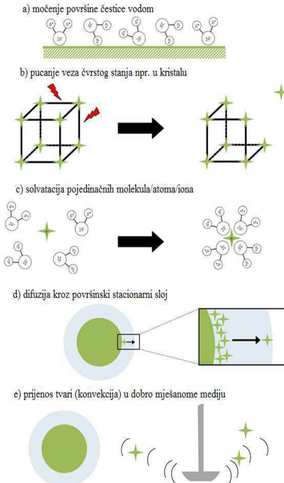
Slika 2. Shematski prikaz pet osnovnih koraka uključenih u proces otapanja čvrste čestice lijeka u dobro mješanom vodenome mediju [preuzeto i prilagođeno prema 22 uz dozvolu Elsevier]
