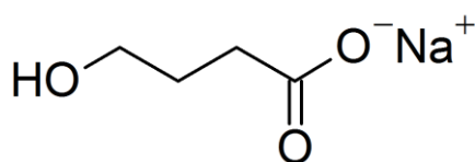
Slika 15. Natrijev oksabat
