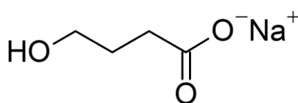
Slika 15. Natrijev oksabat
