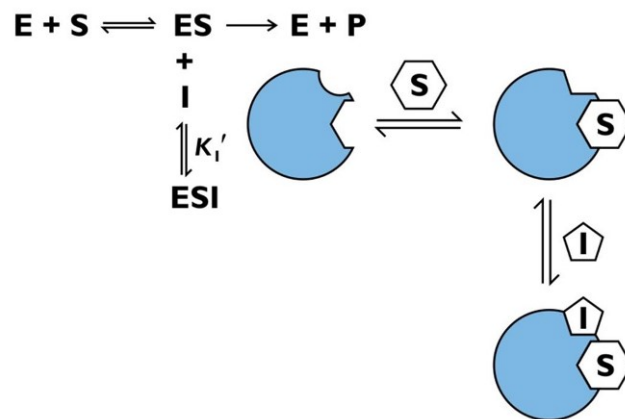
Slika 5. Shematski prikaz akometitivne inhibicije (preuzeto sa: https://www.pmf.unizg.hr )
