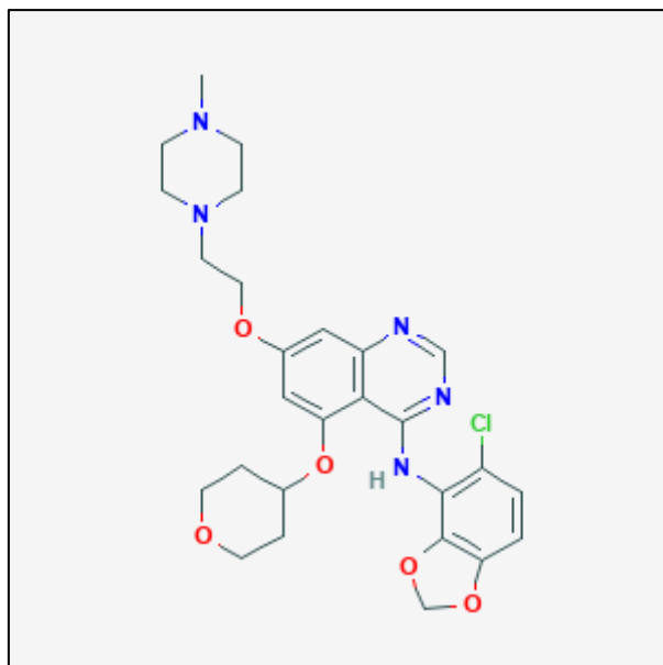
Slika 9. Kemijska struktura saracatiniba (preuzeto iz reference 165).
