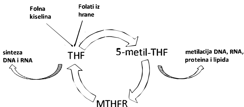
Slika 5. Apsorpcija i biološka aktivacija folata i folatne kiseline te metabolički putevi u kojima sudjeluju folati; THF – tetrahidrofolat; MTHFR – metilentetrahidrofolat reduktaza; 5-metil-THF – 5-metil-tetrahidrofolat
