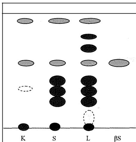
Slika 9a. Kromatogram sterola i triterpenskih kiselina u metanolnim ekstraktima korijena (K), stabljike (S) i lista (L) crvenog likovca ( Daphne cneorum L.). Poredbena tvar: bS – b-sitosterol; Stacionarna faza: Kieselgel 60 F254; Mobilna faza: benzen – aceton (9:1, V/V); Detekcija: klorosulfonska kiselina, zagrijavanje na 105 °C.
