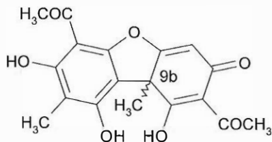
Slika 7. Usninska kiselina
