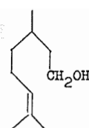
\beta -citronelol
