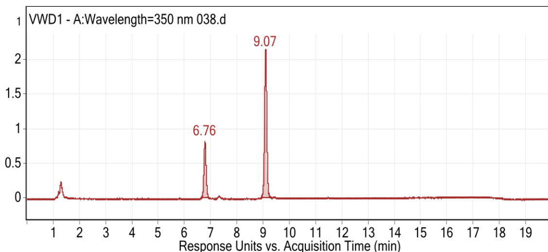
Slika 30. UV kromatogram inkubacijske smjese za 3,7-dihidroksiflavon s dodanim generirajućim sustavom.
