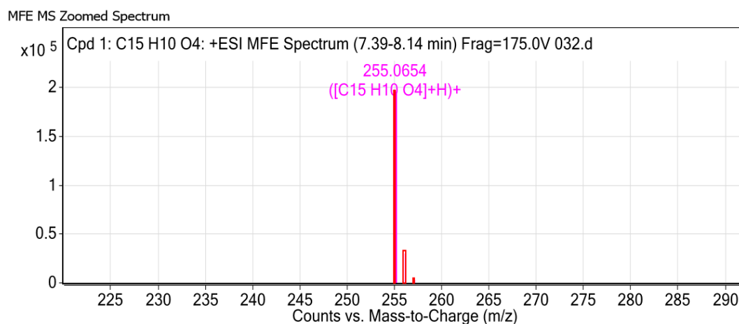
Slika 24. Spektar izdvojenog iona nepoznatog metabolita 7-hidroksiflavona ( m/z = 255,0654 ) u inkubacijskoj smjesi za 7-hidroksiflavin s dodanim generirajućim sustavom.
