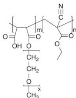
Molekularna struktura poli { \alpha -maleinska kiselina- \omega -metoksi-poli(etilen glikol)-kopolimer-etil cijanoakrilat}
