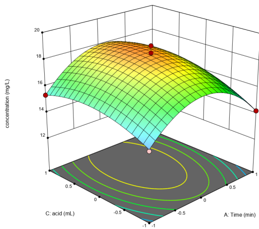
Slika 10. Odzivna površina koncentracije Fe u ovisnosti o udjelu kiseline i vremena soniciranja
