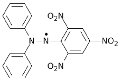
Slika 1.1.1.1.1 Struktura DPPH•
