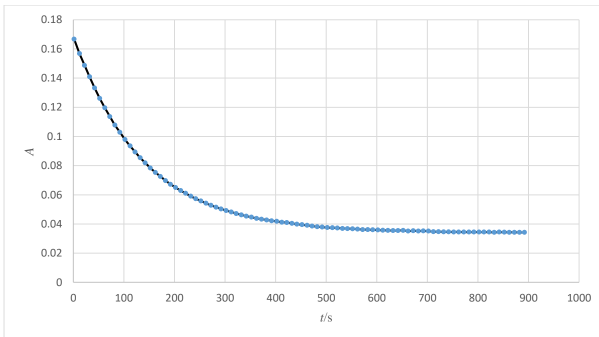
Slika 4.5.3. Ovisnost apsorbancije (A) DPPH• pri 620 nm o vremenu ( t ) za reakciju kvercetina i DPPH• u smjesi otapala dioksan-voda (0,99:0,01, v/v) pri koncentraciji kvercetina 0,001 \text{ mol dm}^{-3} i koncentraciji DPPH• 5 \cdot 10^{-5} \text{ mol dm}^{-3} na temperaturi 25 \text{ }^{\circ}\text{C}
