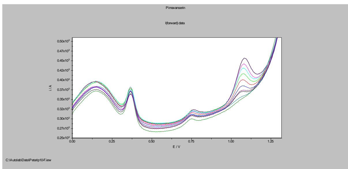
Slika 14. Pravokutnovalni voltamogrami otopina pimavanserina u rasponu koncentracija 5 \times 10^{-7} \text{ mol/dm}^3 (tamno zelena linija) – 1 \times 10^{-5} \text{ mol/dm}^3 ( tamno plava linija), i levodope pri konstantnoj koncentraciji ( c=2 \times 10^{-5} \text{ mol/dm}^3 ), dobiven pri optimalnim uvjetima.
