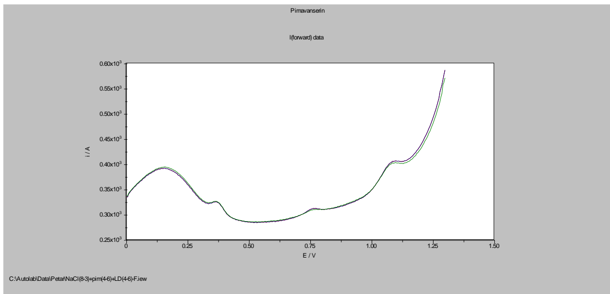
Slika 21. Pravokutnovalni voltamogrami levodope ( c=4 \times 10^{-6} \text{ mol/dm}^3 ), pimavanserina ( c=4 \times 10^{-6} \text{ mol/dm}^3 ) i natrijeva klorida koncentracije 4 \times 10^{-3} \text{ mol/dm}^3 (plava krivulja) i 8 \times 10^{-3} \text{ mol/dm}^3 (zeleno krivulja) pri optimalnim uvjetima.
