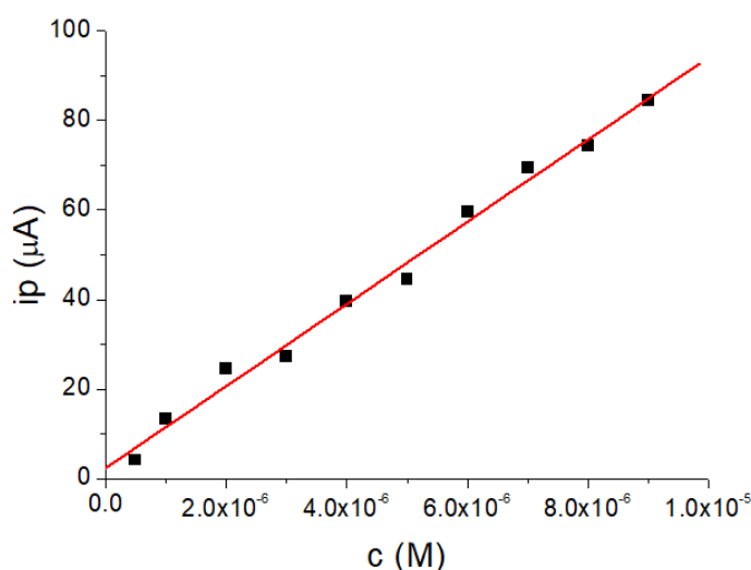
Slika 15. Prikaz ovisnosti izmjerenih jakosti struja pimavanserina o njegovoj koncentraciji ( 5 \times 10^{-7} M – 9 \times 10^{-6} M), dobivenih upotrebom modificirane elektrode SQW voltametrijom pri f=75 Hz, E=20 mV i dE=4 mV, nakon akumulacije tijekom 60 s pri 0 V.
