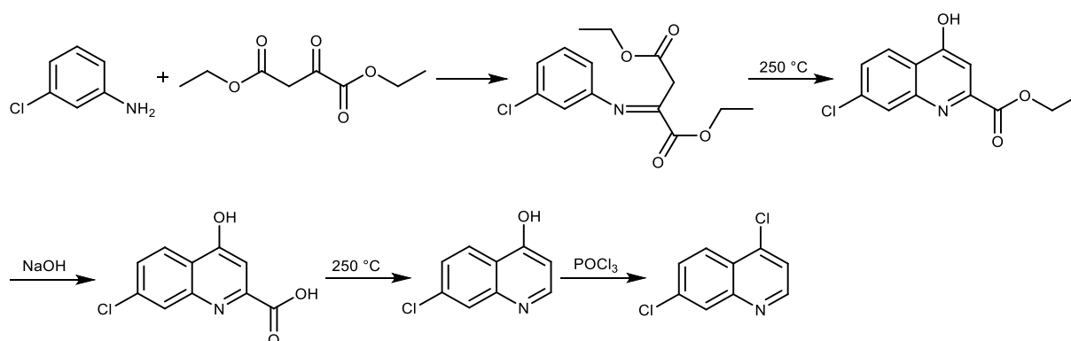
Shema 5. Sinteza 4,7-diklorkinolina prema Metodi 1
