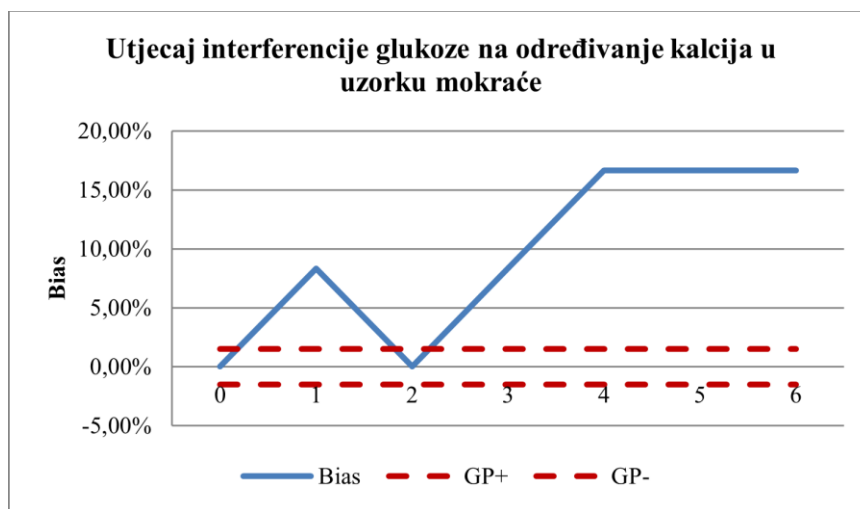
Slika 23 Grafički prikaz utjecaja interferencije glukoze na određivanje kalcija u uzorku mokraće
