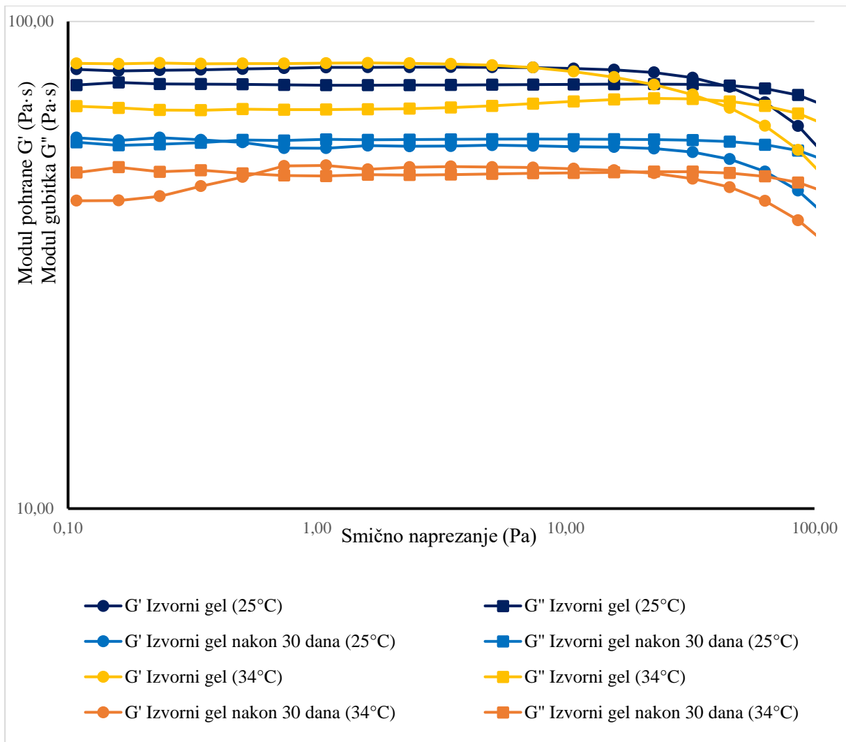
Slika 14. Grafički prikaz ovisnosti modula pohrane G' i modula gubitka G'' o smičnom naprezanju za izvorni gel na 25 °C i 34 °C neposredno nakon izrade formulacije te nakon 30 dana skladištenja.
